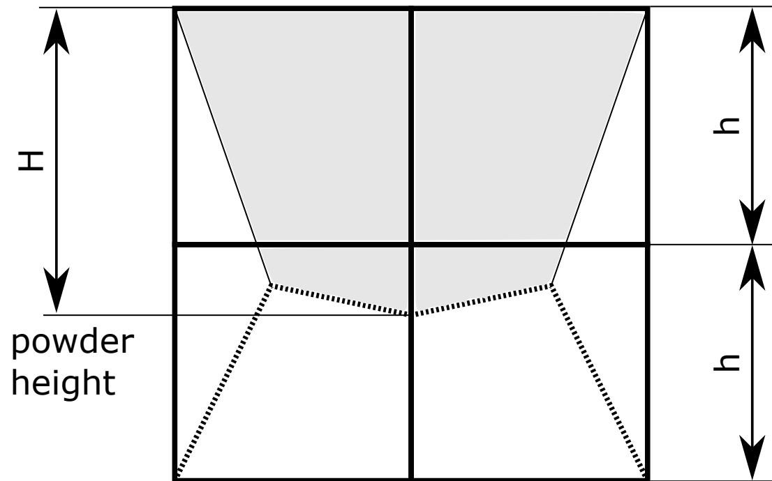
fixed layer height increment
